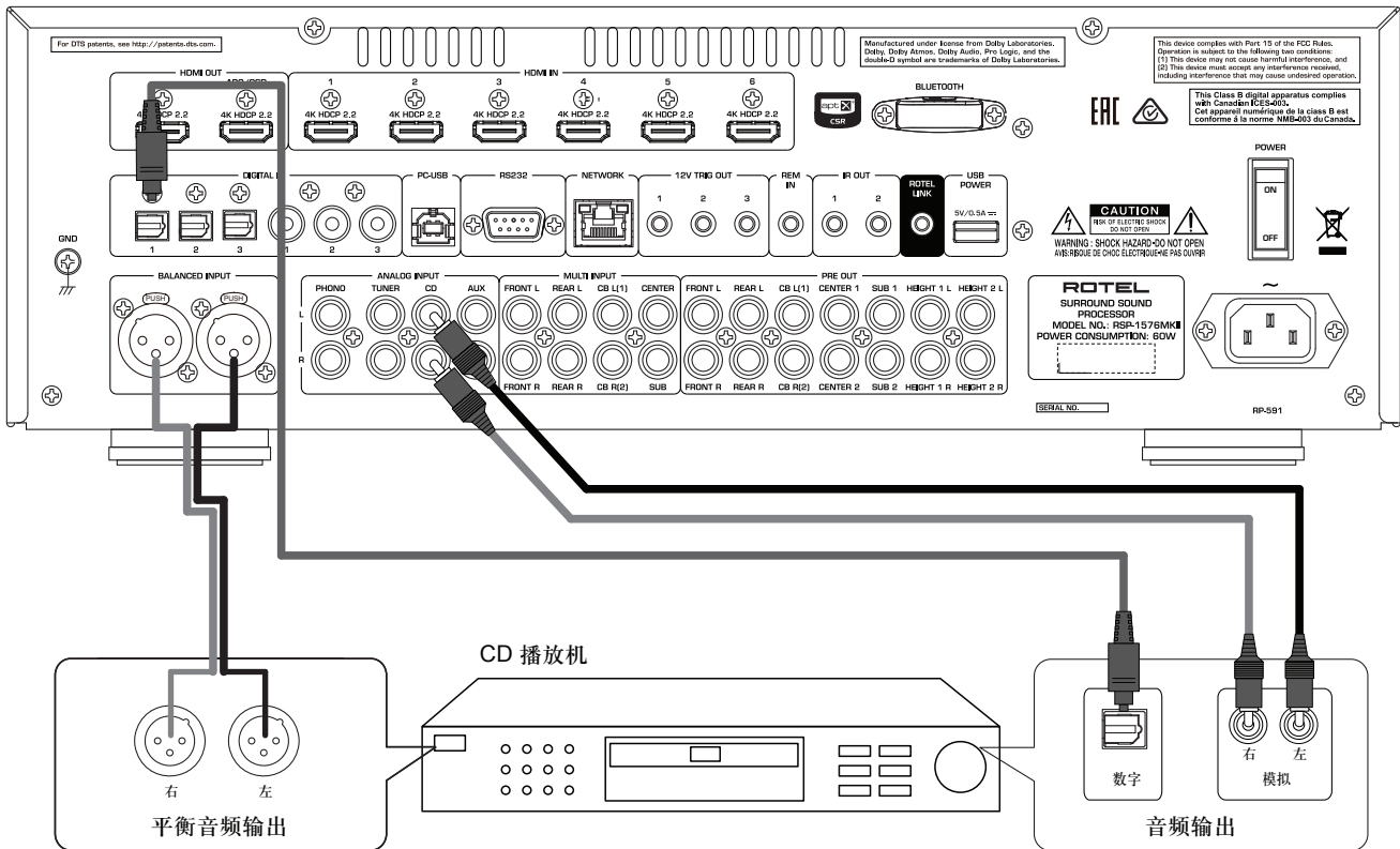
图7： CD播放机连接
