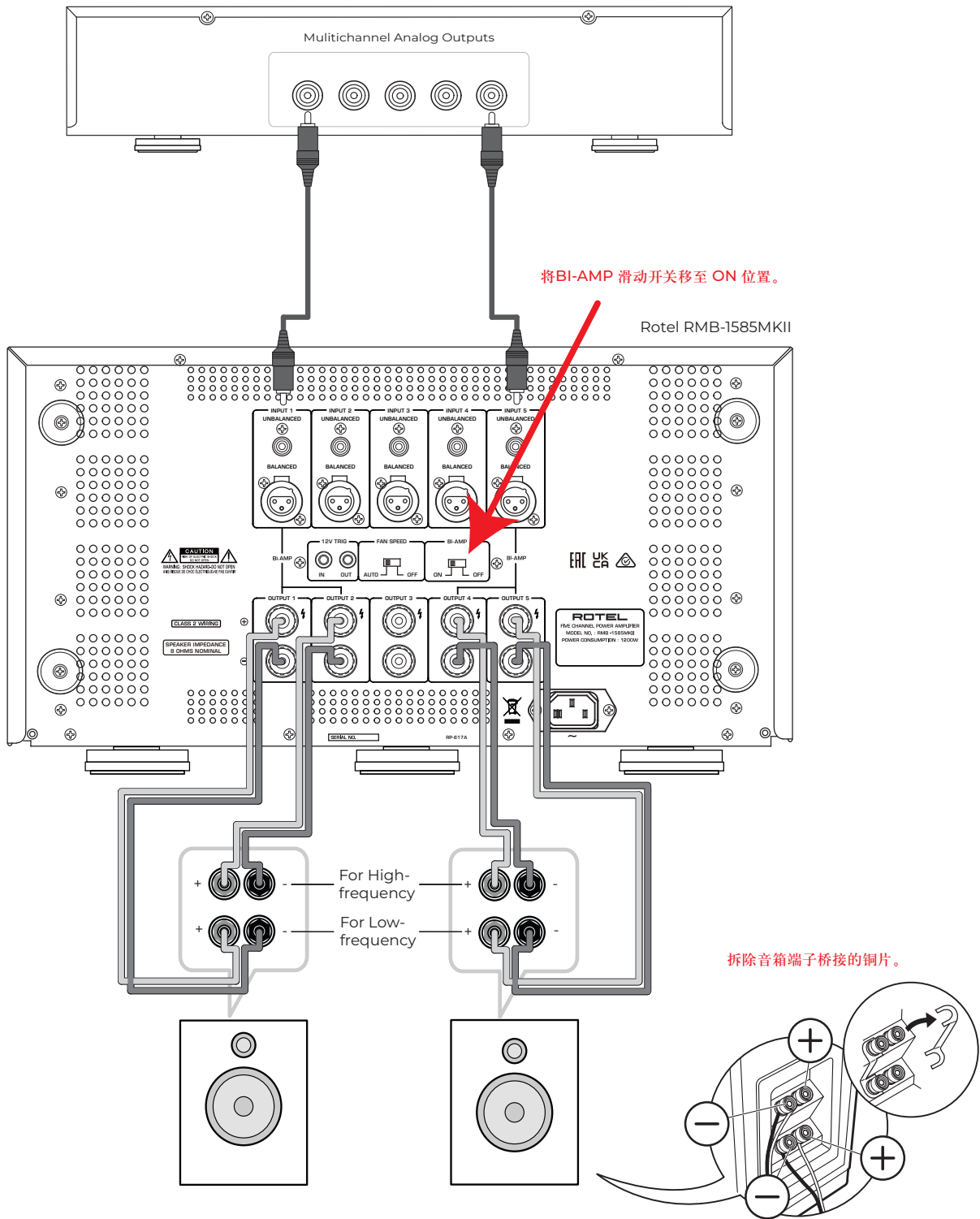
图 4: 双功放(Bi-Amping)连接
