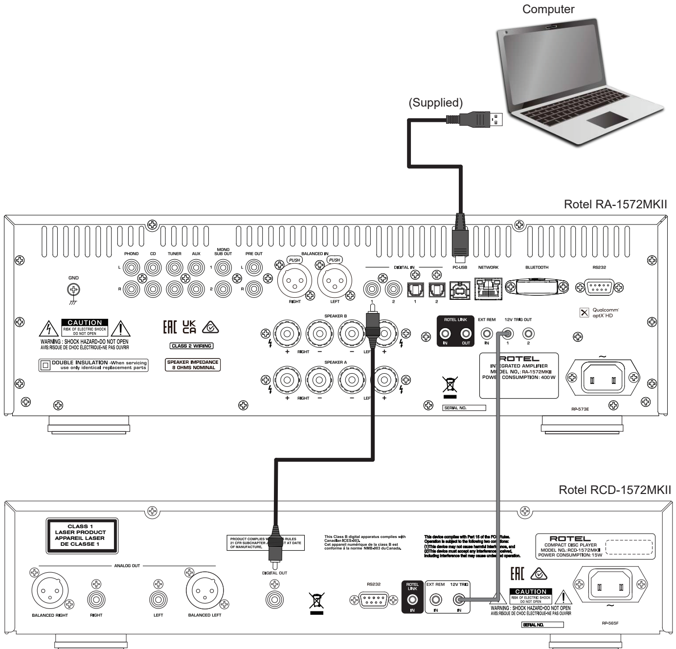
Figure 4 : Digital Input and 12 Volt Trigger Out Connections Entrées numériques et Branchements des sorties trigger 12 V Anschlussdiagramm (Digitaleingänge, 12V-Trigger-Ausgänge) Entrada Digital y Conexiones de Salida para Señal de Disparo de 12 Voltios Digitale ingangen en 12V-triggeruitgangen Collegamenti ingressi digitali e segnali Trigger 12 V Anslutningar för digitala ingångar och 12-volts styr signaler Цифровой вход и выход 12-В триггерного сигнала
