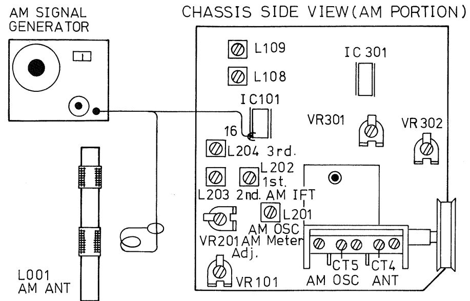
Fig. 1. AM IF and RF Alignment Hook-Up Abb. 1. AM-ZF und HF-Abgleich Fig. 1. Aligement AM IF et HF
