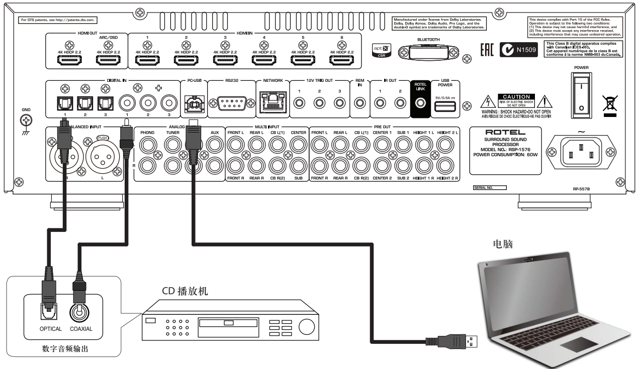
图4: 数字音频和PC-USB连接
