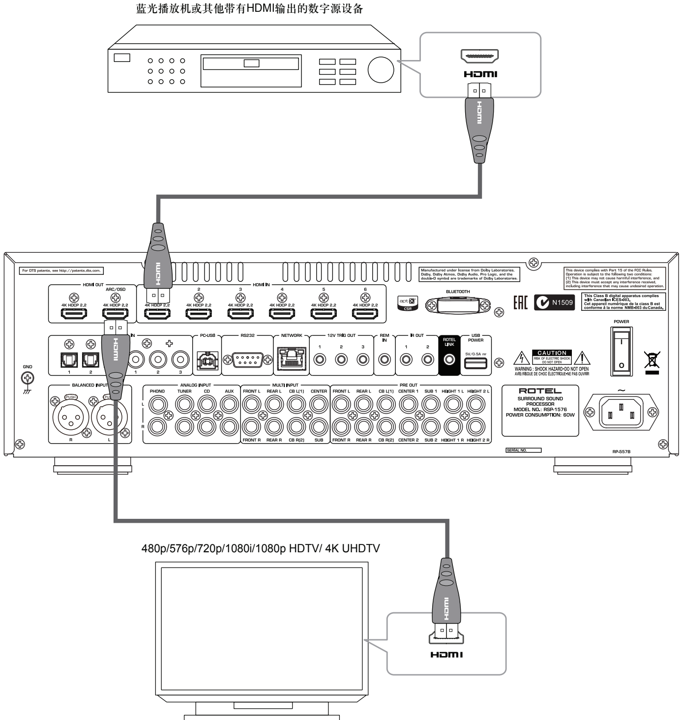
图10: 后置HDMI连接
