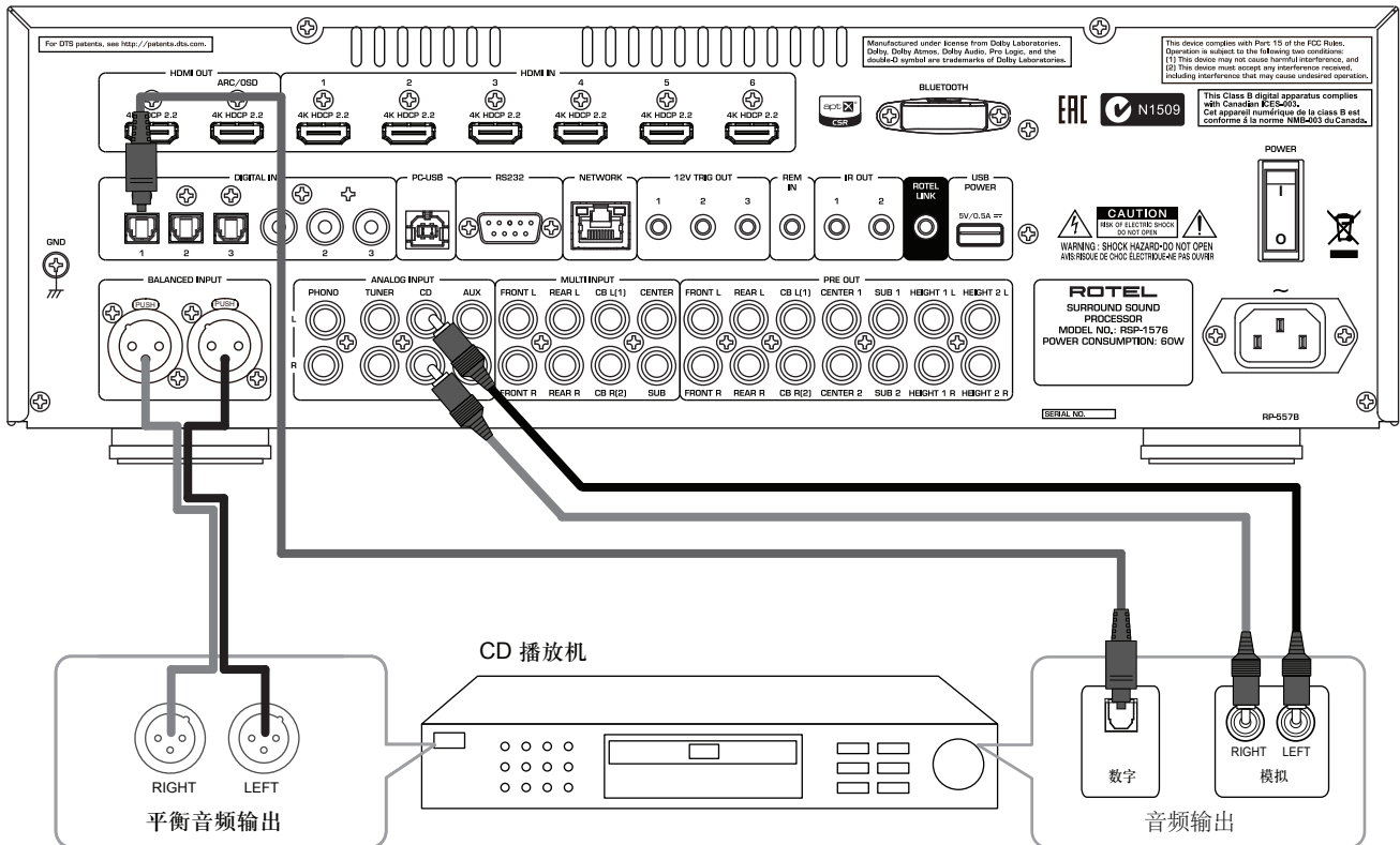
图7： CD播放机连接
