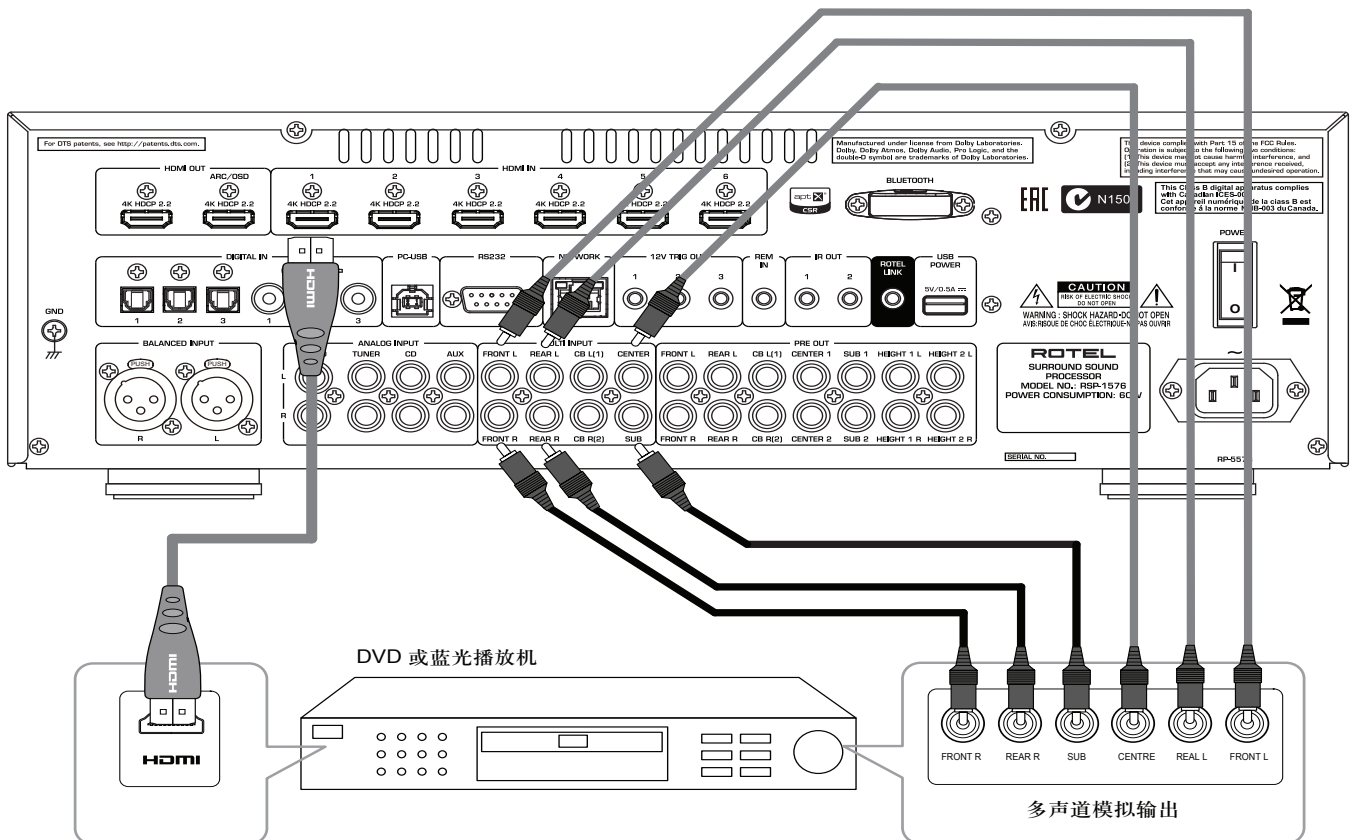
图5: 蓝光机和视频播放机连接
