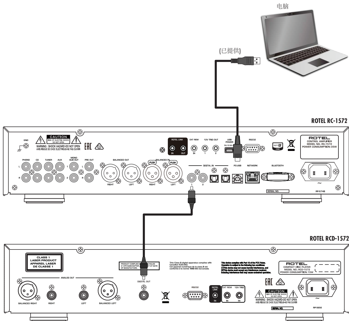
图 5: 数字输入连接
