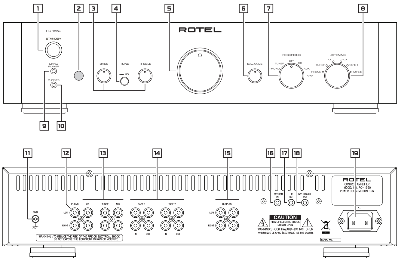
Figure 1: Controls and Connections Commandes et branchements Bedienelemente und Anschlüsse Controles y Conexiones De bedieningsorganen en de aansluitingen Controlli e connessioni Kontroller och anslutningar Органы управления и разъемы
